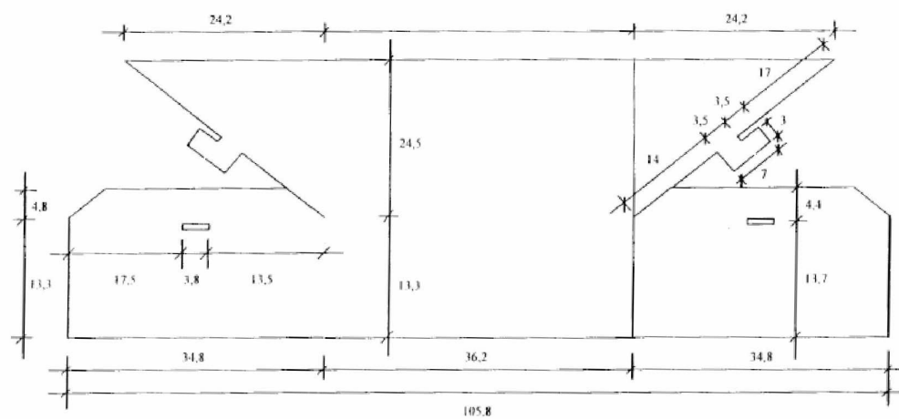
PLANTA DA CABINA DE VOTAÇÃO COLAS EM CM
